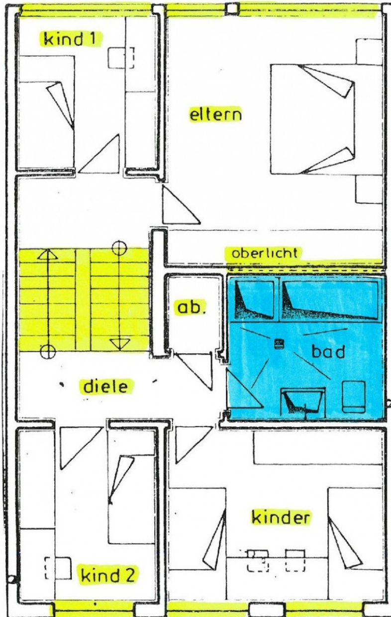
14 Obergeschoss Grundriss Keine Gewähr
